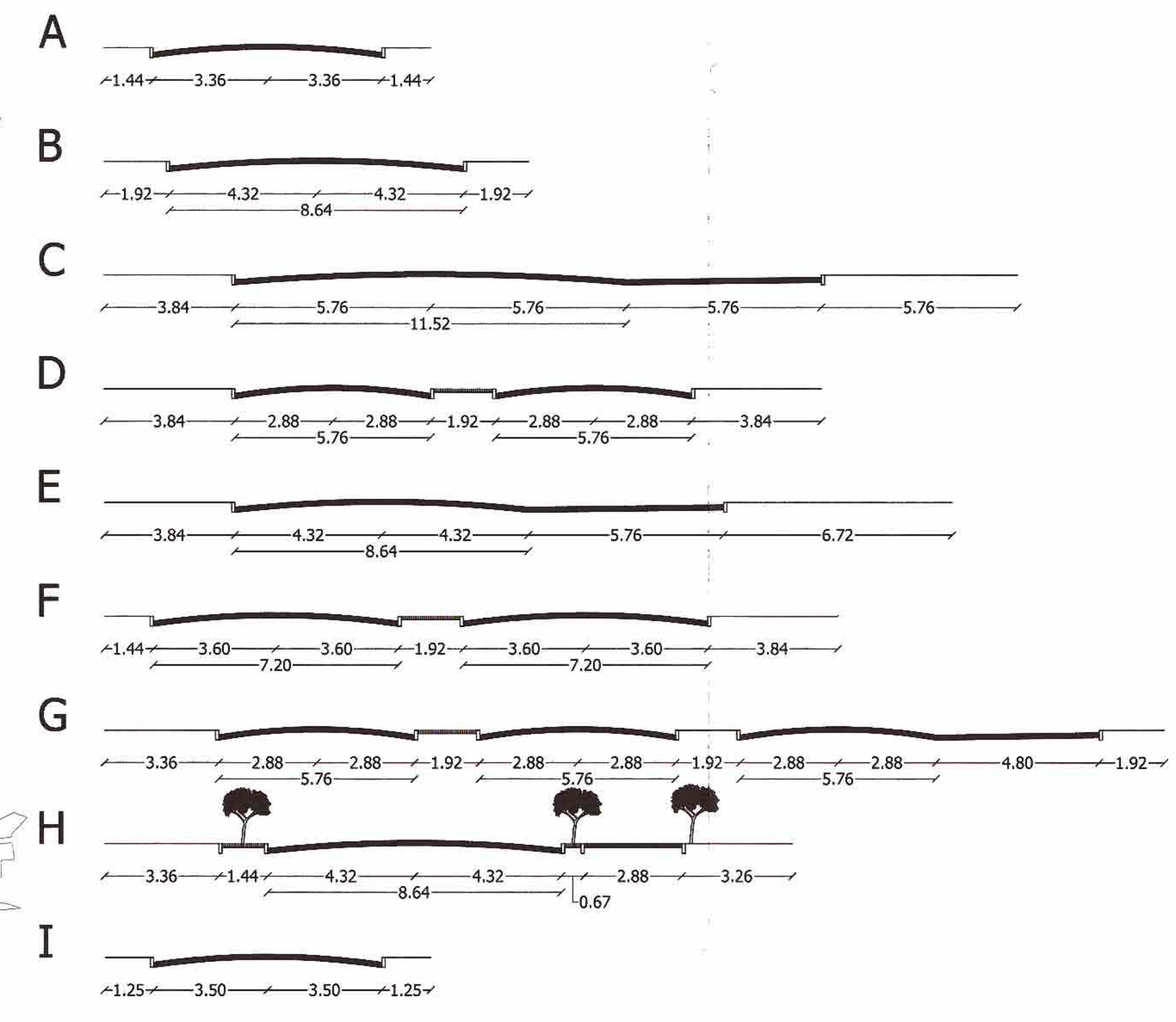
Schemi SEZIONI STRADALI esistenti e di progetto
